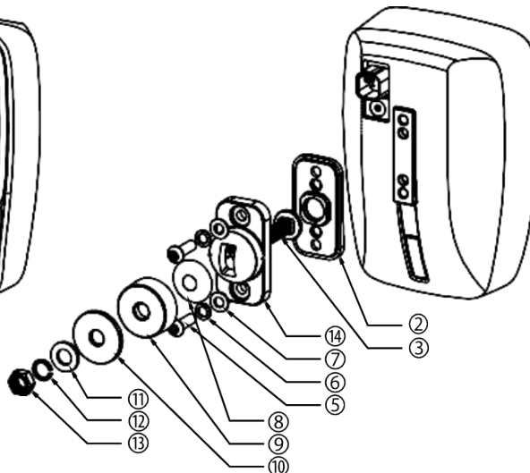
MONTAGE A L'ARRIÈRE GAUCHE & DROIT
