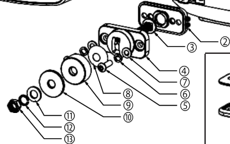
MONTAGE A L'ARRIÈRE GAUCHE & DROIT
